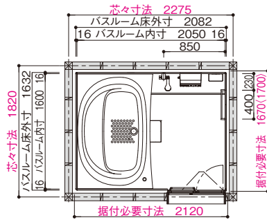
平面図・立面図
