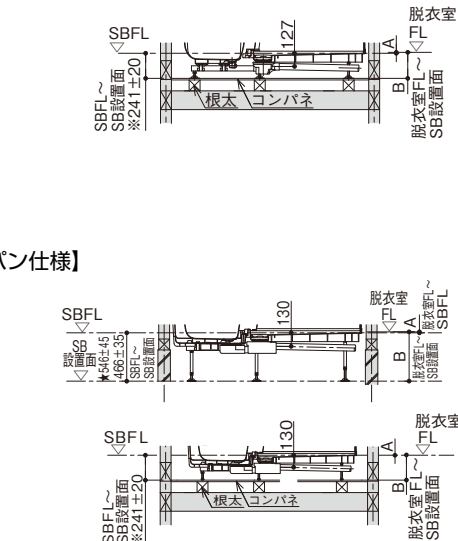
階上設置の場合
