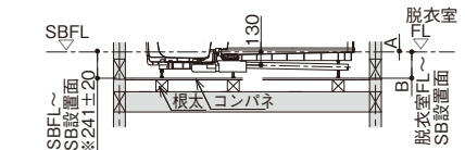
階上設置の場合
