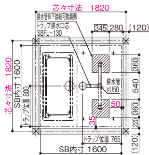
排水管落とし可能位置図
