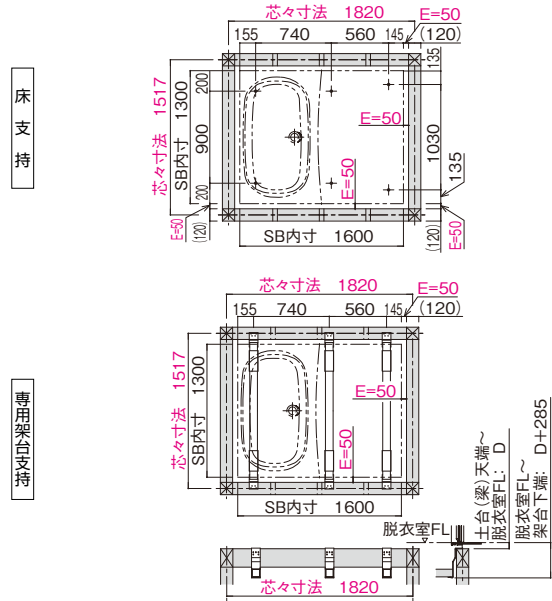
床支持位置図
