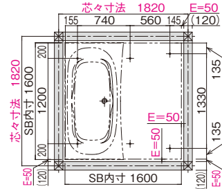
床支持位置図
