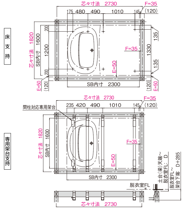
床支持位置図
