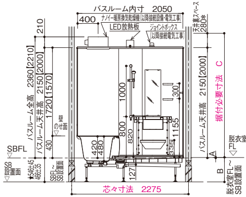
【浴槽パンなし仕様】
