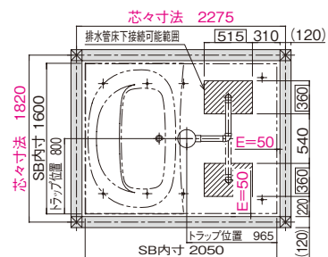
排水管落とし可能位置図
