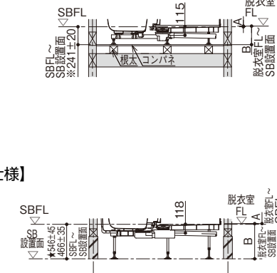
階上設置の場合
