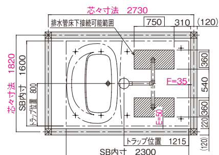
排水管落とし可能位置図
