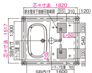
排水管落とし可能位置図
