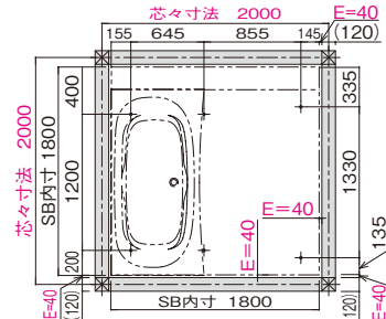
床支持位置図
