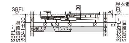
階上設置の場合
