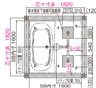
排水管落とし可能位置図
