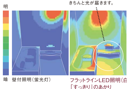
◎浴室内部照度分布図
