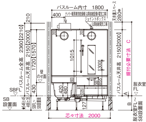
【浴槽パンなし仕様】
