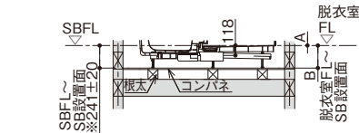
階上設置の場合
