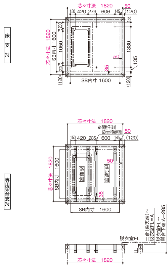
床支持位置図
