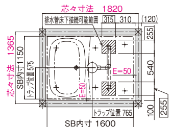
排水管落とし可能位置図
