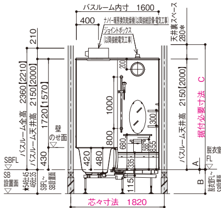
【浴槽パンなし仕様】
