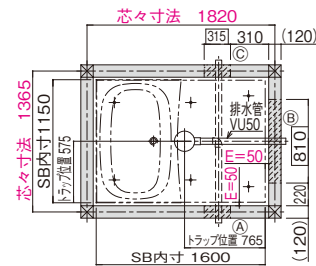
排水管けり出し可能位置図
