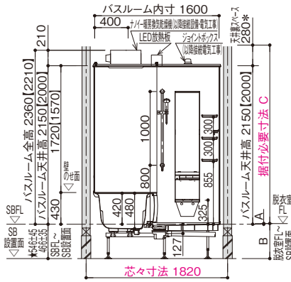
【浴槽パンなし仕様】
