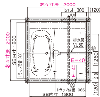
排水管けり出し可能位置図
