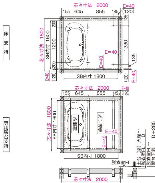
床支持位置図
