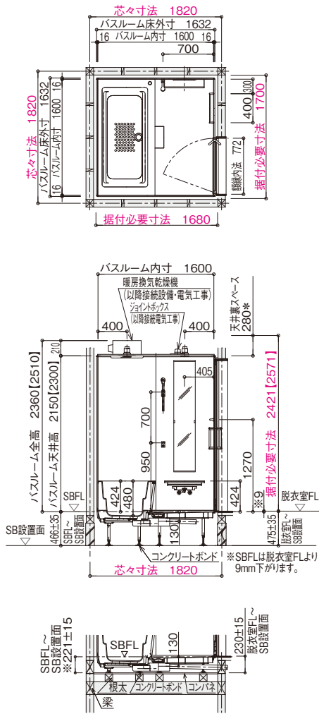
平面図・立面図
