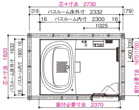
【浴槽パンなし仕様】
