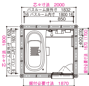
平面図・立面図
