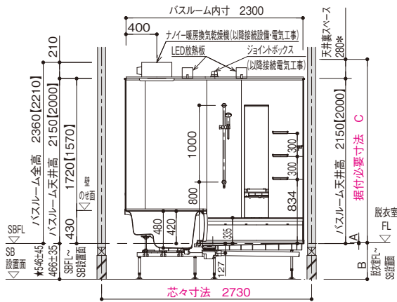
【浴槽パンなし仕様】
