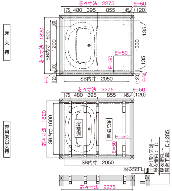
床支持位置図
