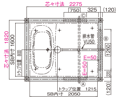
排水管けり出し可能位置図
