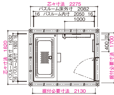
平面図・立面図
