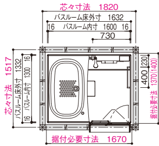
平面図・立面図
