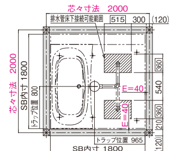
排水管落とし可能位置図
