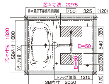
排水管落し可能位置図
