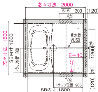
排水管けり出し可能位置図
